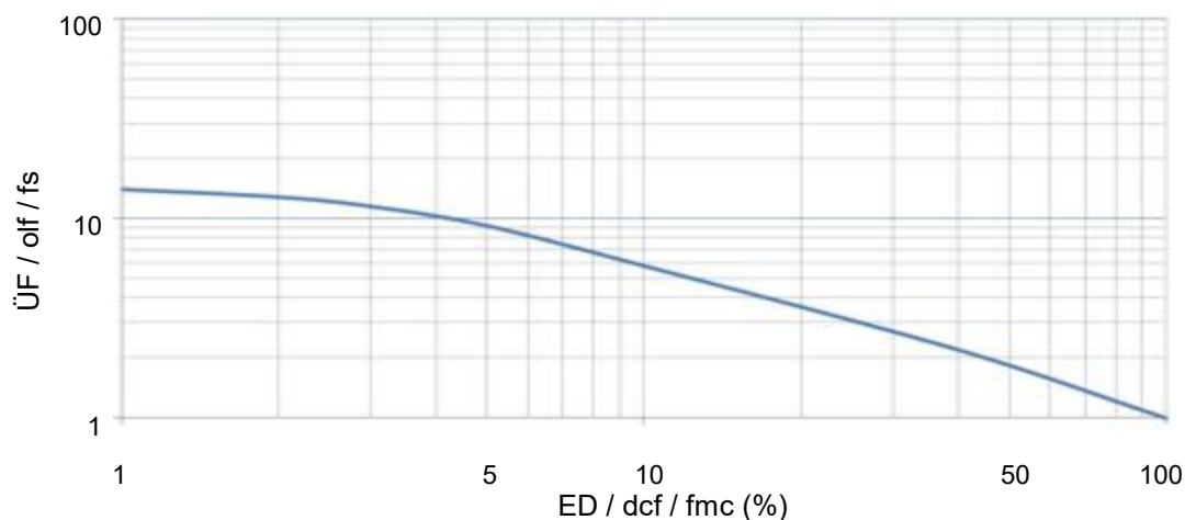
Überlastfaktor ( ÜF ) in Abhängigkeit der Einschaltdauer ( ED ) für Zykluszeit = 120 s Overload factor ( olf ) in dependence of duty cycle factor ( dcf ) for total cycle time = 120 s Facteur de surcharge ( fs ) en rapport avec le facteur de mise en circuit ( fmc ) pour une durée de cycle = 120 s
